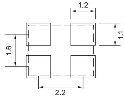
推奨ランドパッド/Solder Pad Layout
